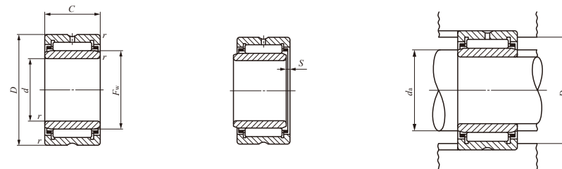
NA49 NA48
